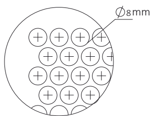
DETTAGLIO GRIGLIA FORI Ø 8mm
